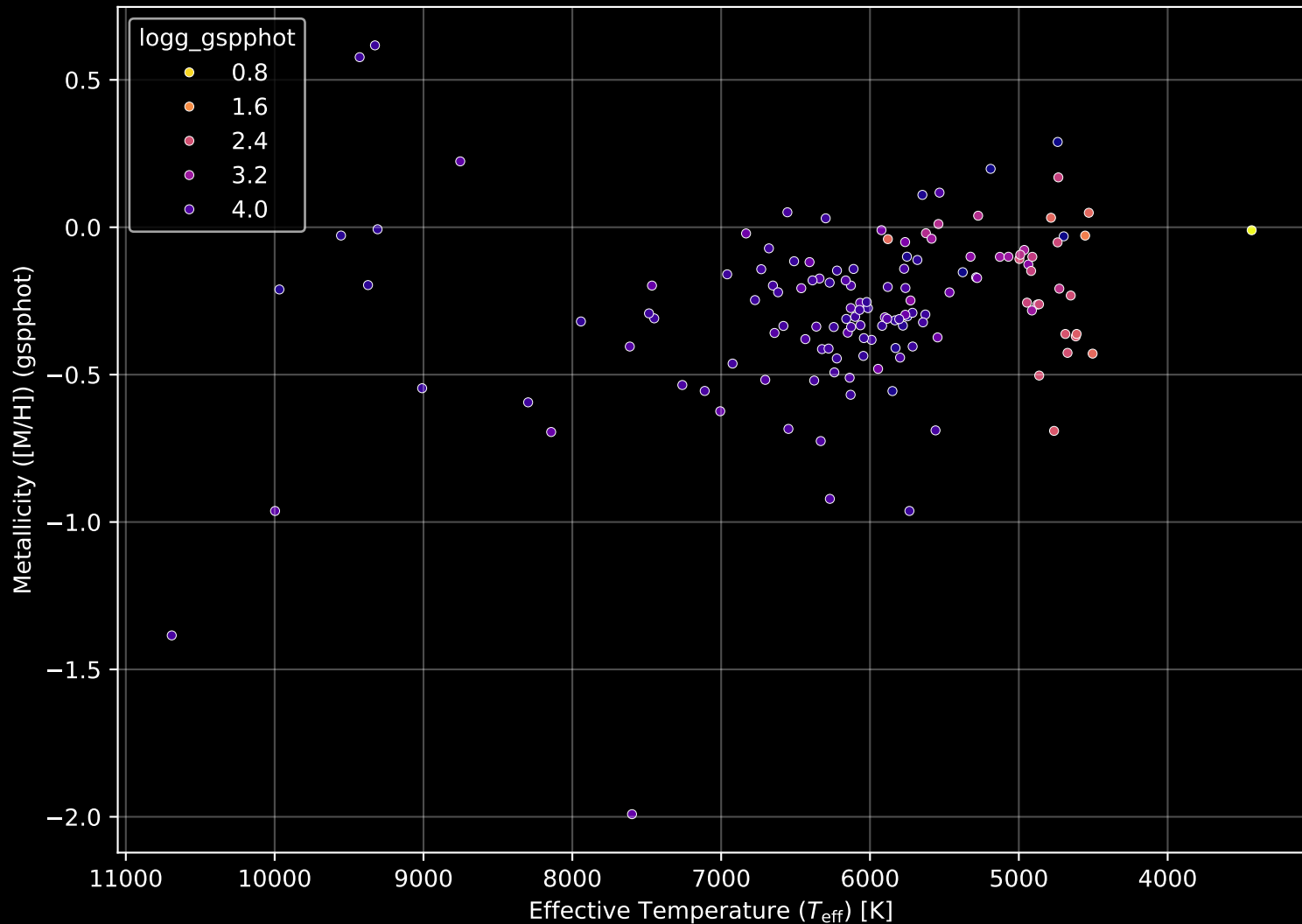
GALAH DR4 Field: [2545] Stellar Population Parameters (n= 139)
