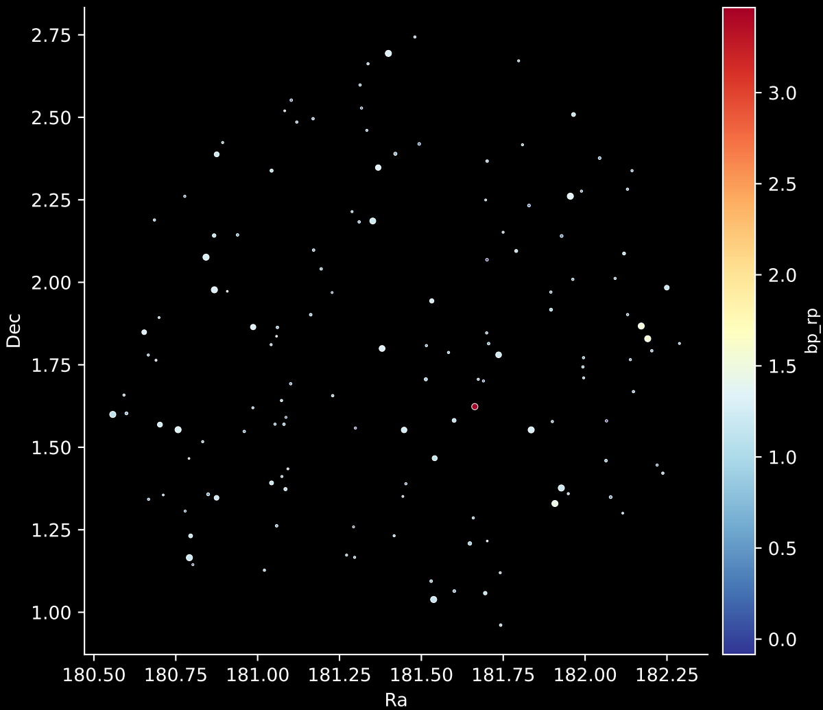
GALAH DR4 Field: [2545] Stars: 139
