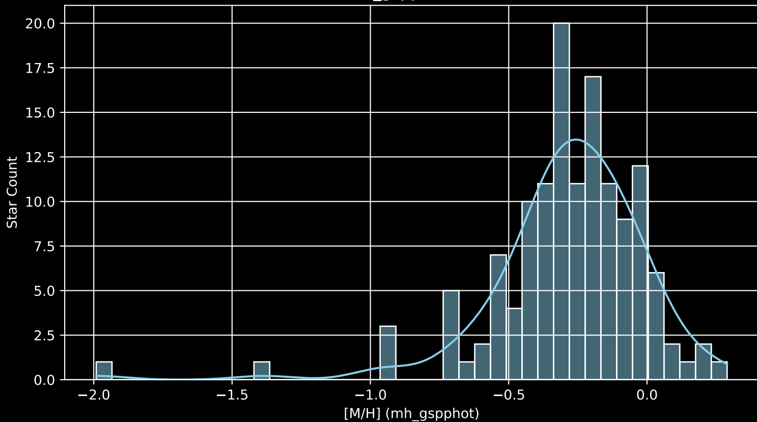
GALAH DR4 Field: [2545] [M/H] (mh_gspphot) (n= 137)
