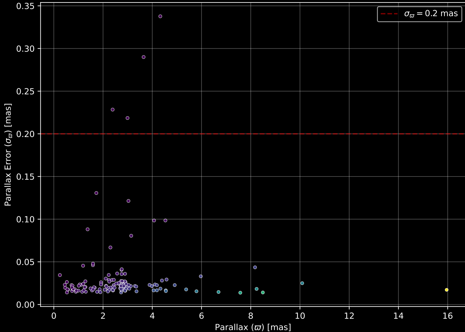
GALAH DR4 Field: [2545] Parallax Quality (n= 139)
